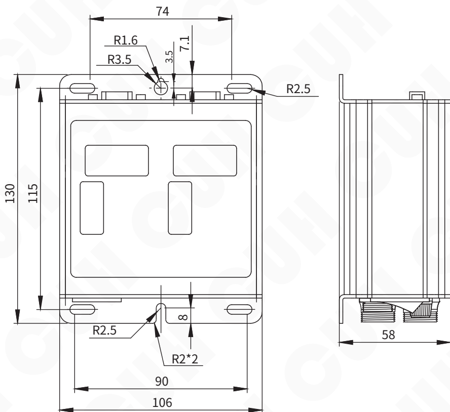
智能数字振动送料控制器SDVC22-S外形尺寸 (单位: mm)
