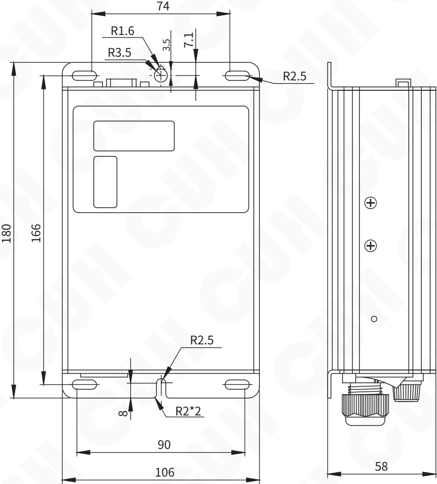
智能数字振动送料控制器SDVC20-L外形尺寸（单位：mm）
